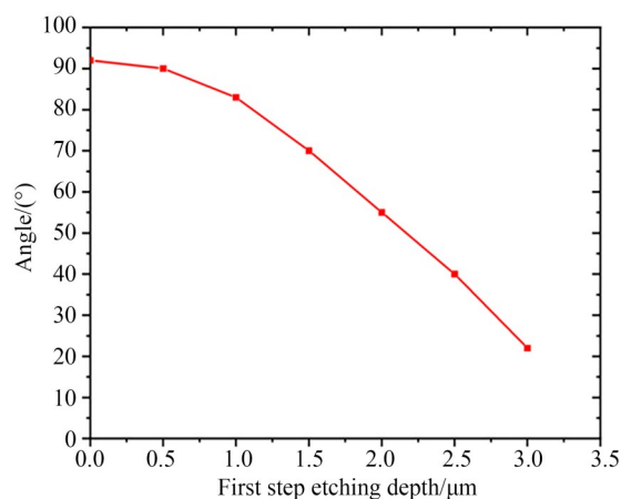
(a) 第一步不同刻蚀深度与上壁和侧壁夹角的关系,夹角位置如图2(e)所示
