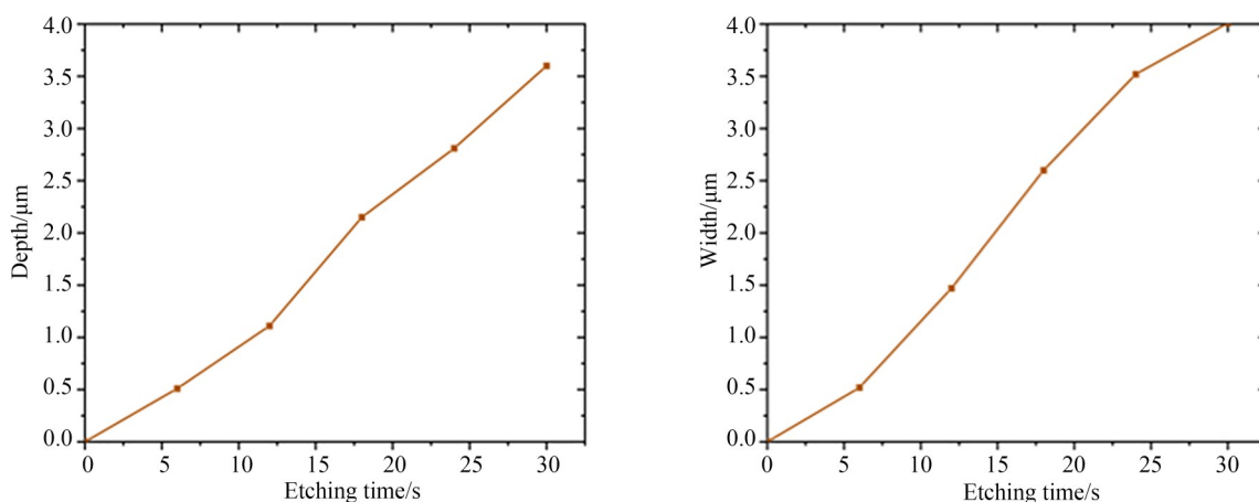
图5 各向同性刻蚀时间与高度和宽度的关系
