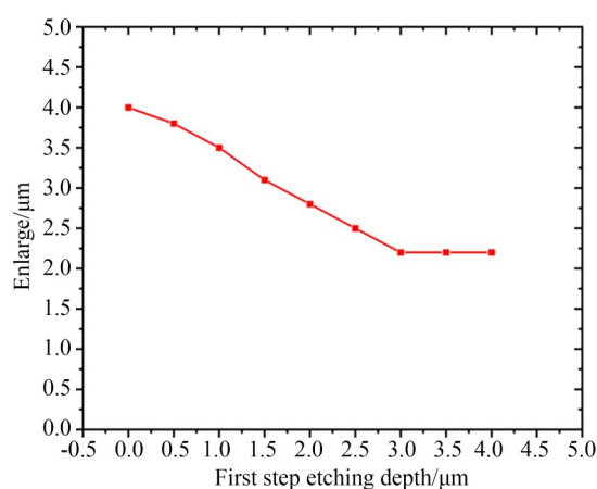
(b) 第一步不同刻蚀深度与各向同性刻蚀下增大的微孔直径的关系
