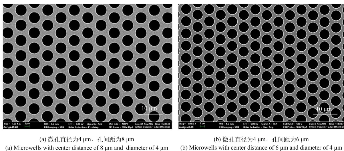
图 1 两步刻蚀法制备的微孔正视图(微孔呈正三角形分布)
